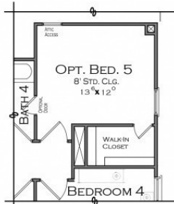
OPTIONAL BED 5 OPTION ADDS 223 SQ. FT. OPTIONAL DOOR
